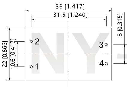
底视图
