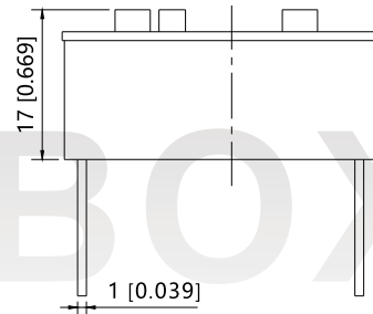
正视图
