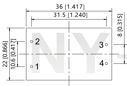
底视图
