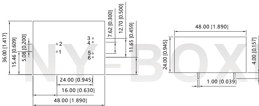
底视图
