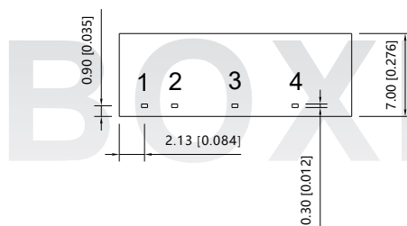
底视图
