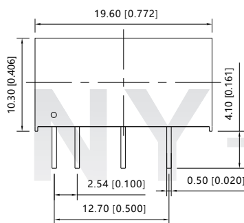
前视图
