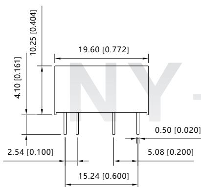
前视图
