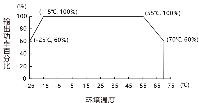
温度降额曲线
