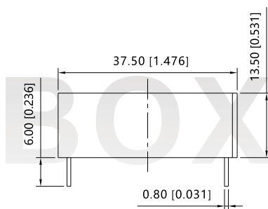
前视图
