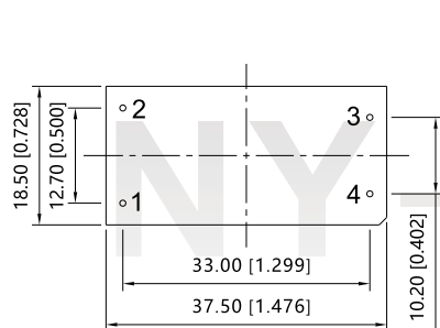
底视图
