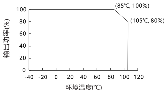
温度曲线图
