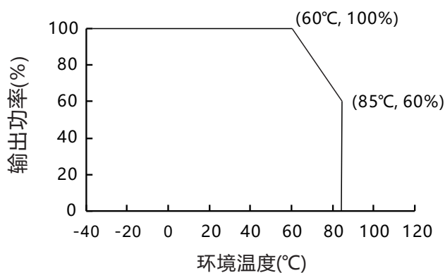
温度曲线图
