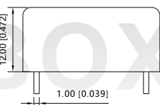
前视图
