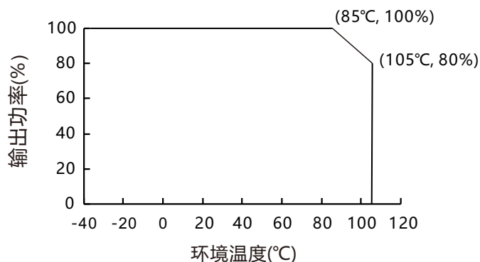
温度曲线图
