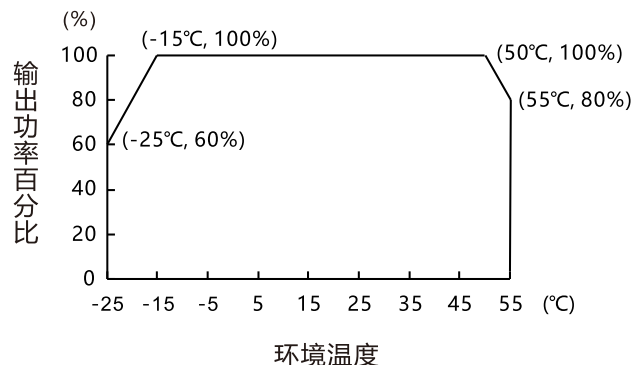
温度降额曲线 输入电压: 85~264VAC 100~375VDC
