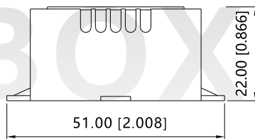
正视图
