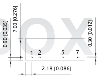
底视图
