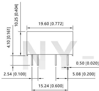
前视图
