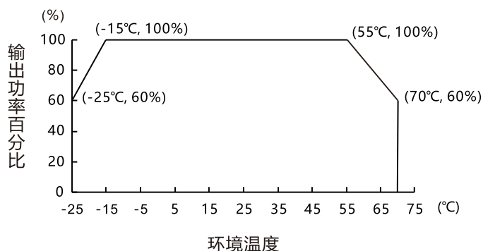
温度降额曲线 输入电压：85~264VAC 100~375VDC
