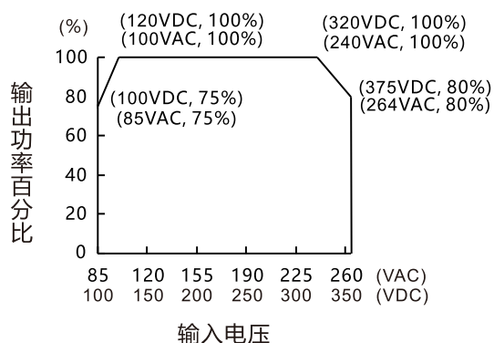
输入电压降额曲线 (工作温度：25℃)
