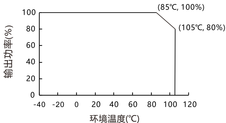
温度曲线图
