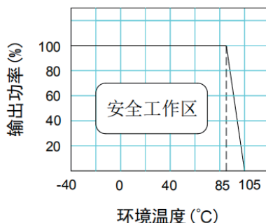
温度曲线图
