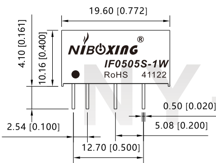
前视图
