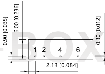
底视图
